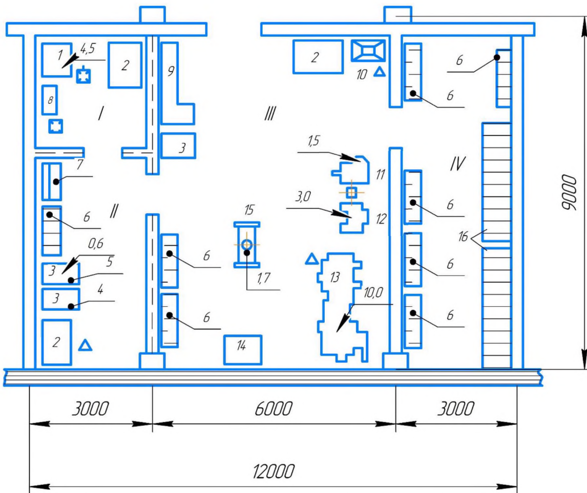
Рис. 29. Планировка участка отдела главного механика по типовому проекту таксомоторного парка на 325 автомобилей (Гипроавтотранс):
